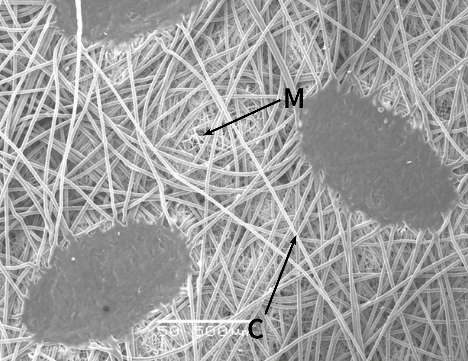
ЕЛЕКТРОННА СКАНУЮЧА МІКРОФОТОГРАММА ОСНОВНОГО МАТЕРІАЛУ СММС ЗБІЛЬШЕННЯ X 500
