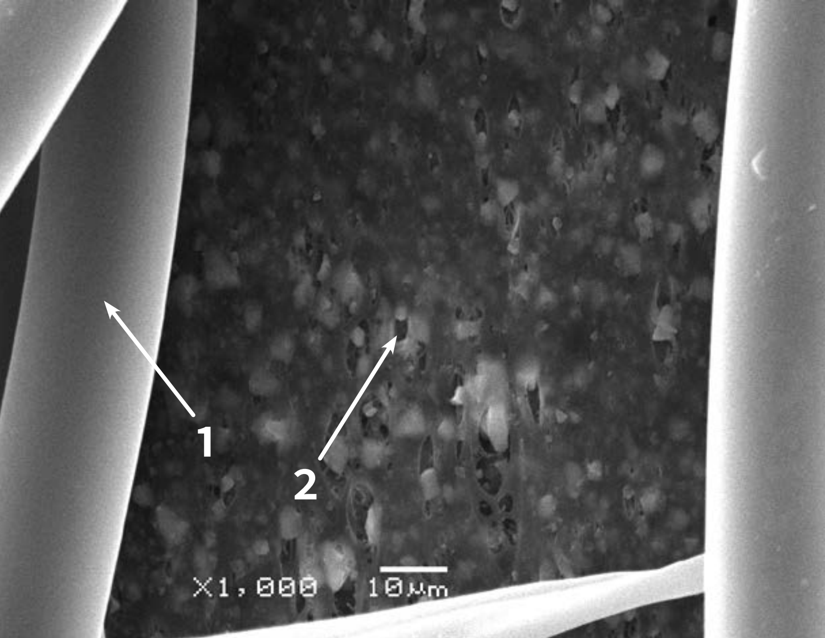
ЕЛЕКТРОННА СКАНУЮЧА МІКРОФОТОГРАММА ПОСИЛЮЮЧОЇ МЕМБРАНИ ЗБІЛЬШЕННЯ X 1000
